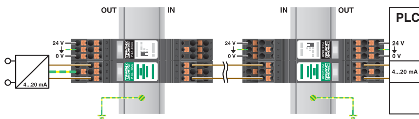
rysunek aplikacji
