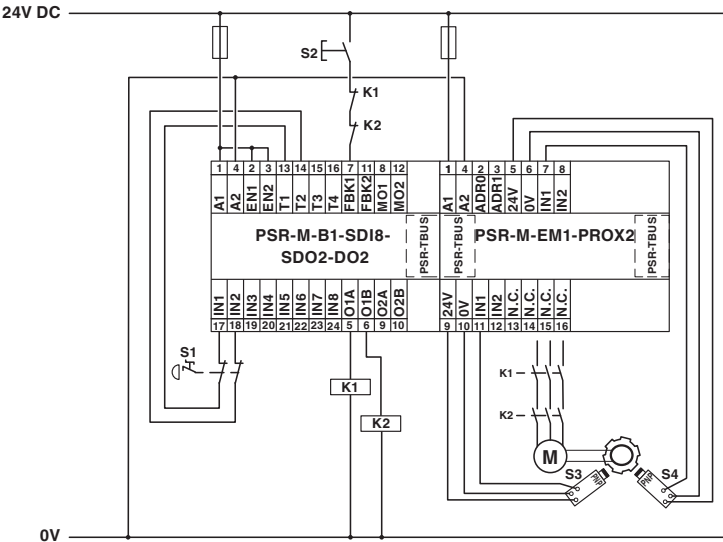
rysunek aplikacji
