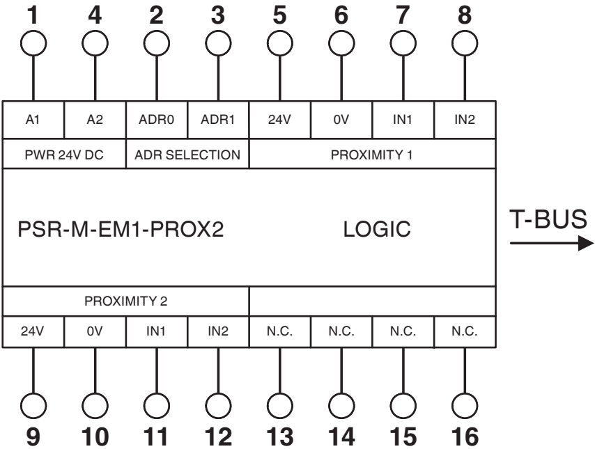
Schemat blokowy
