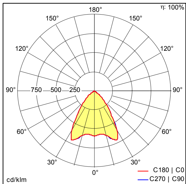
D43023AA_MIRL_LAY_LED3800-840_M600Q_EVG_WH.Idt
