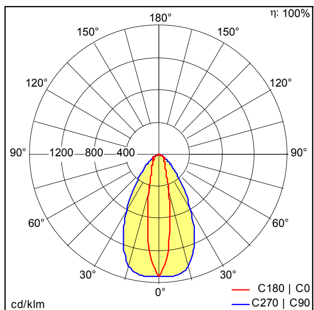
D43653AA_TECTON_C_LED10000-840_L2000_NB_LDE_WH.Idt
