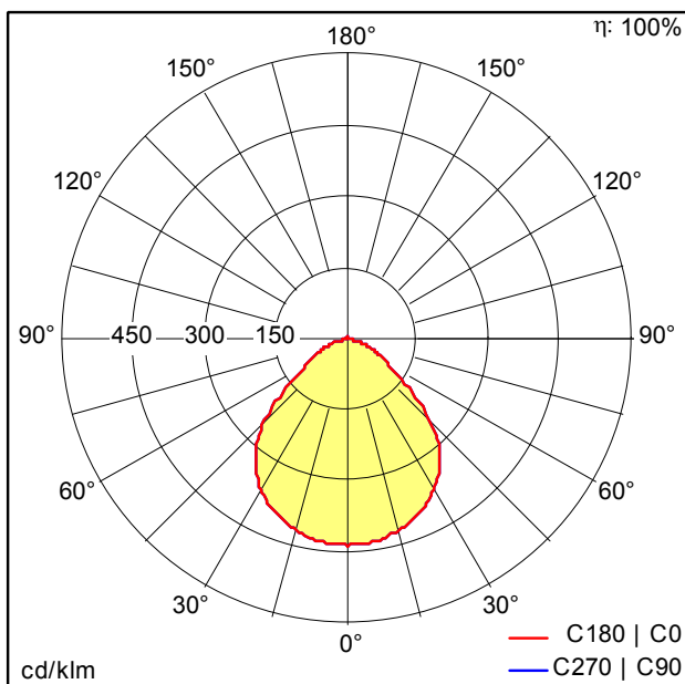
D37457AA_ONDA2_P_LRO_D1150_LED16000-830.Idt
