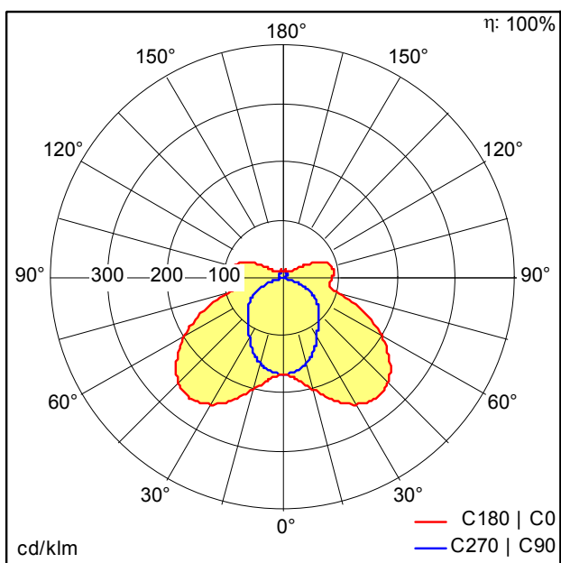
D45907_AMP_L_4600-840_PC_WB_EVG.Idt
