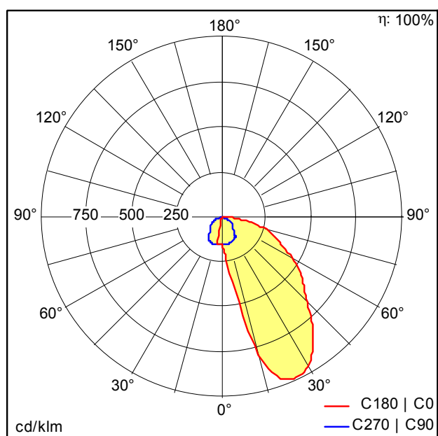
D34983AA_TECTON_C_LED7400-865_L2000_WW_LDE_WH.Idt
