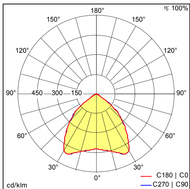
D43022AA_MIRL_LAY_LED3800-840_M600Q_WB_EVG_WH.Idt
