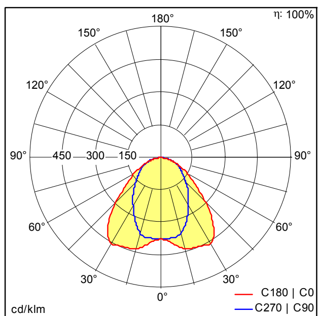
D41246AA_TECTON_C_LED5200-830_L1000_VWB_LDE_WH.Idt
