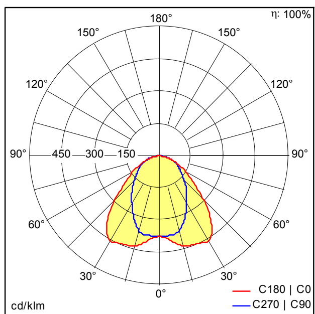
D41246AA_TECTON_C_LED8000-840_L1500_VWB_LDE_WH.Idt
