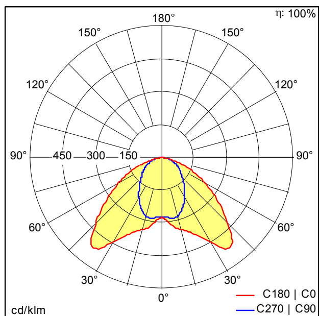
D41186AA_TECTON_C_LED7400-840_L2000_WSB_LDE_WH.Idt
