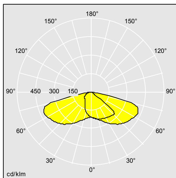
TL_IP12L50NR740.Idt
