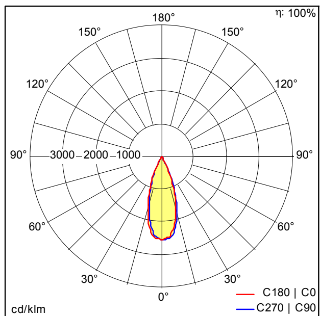
TE_LUCA_M_38°_940.ltd
