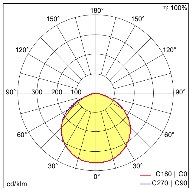
TE_LEONIE_VARIOFLEX_40W_840_FLEX1.ltd
