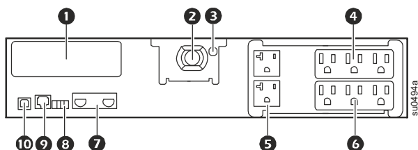
Zasilacz 3000 VA niskonapięciowy
