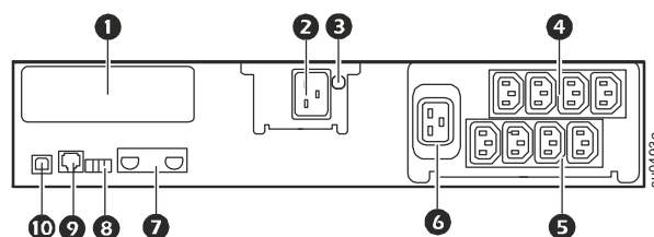
Zasilacz 2200/3000 VA wysokonapięciowy
