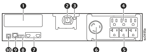
Zasilacz 3000 VA niskonapięciowy
