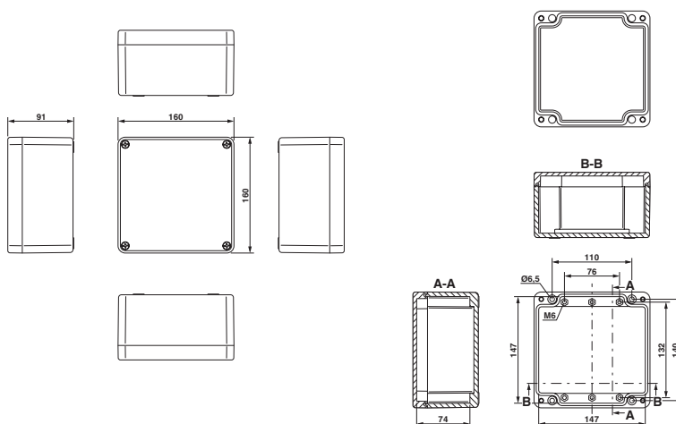
Rysunek wymiarowy
