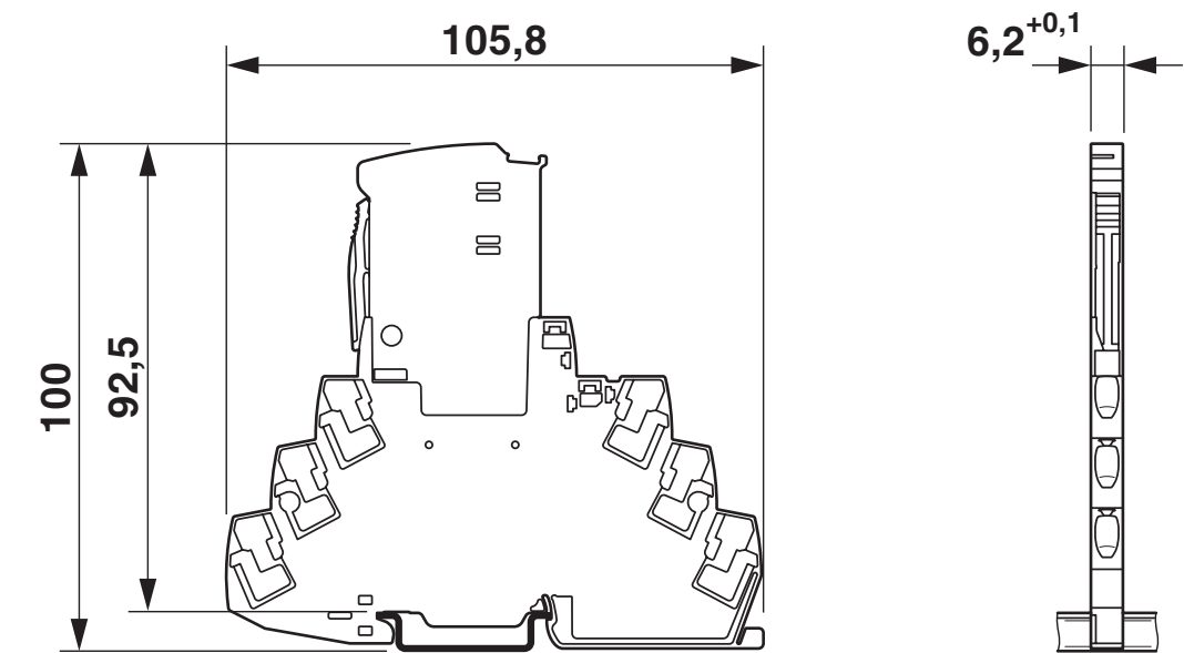
Rysunek wymiarowy
