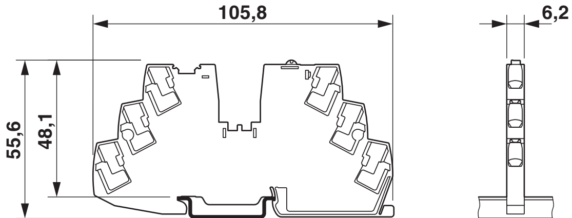
Rysunek wymiarowy
