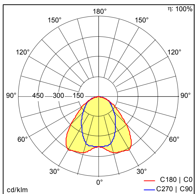
D41246AA_TECTON_C_LED5200-840_L1000_VWB_LDE_WH.Idt
