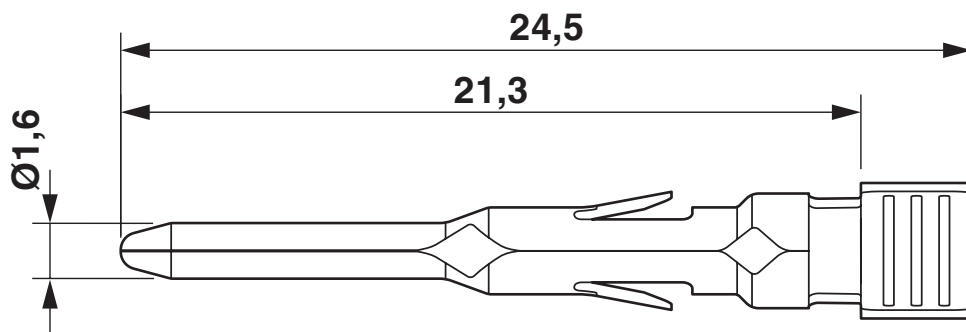
Rysunek wymiarowy
