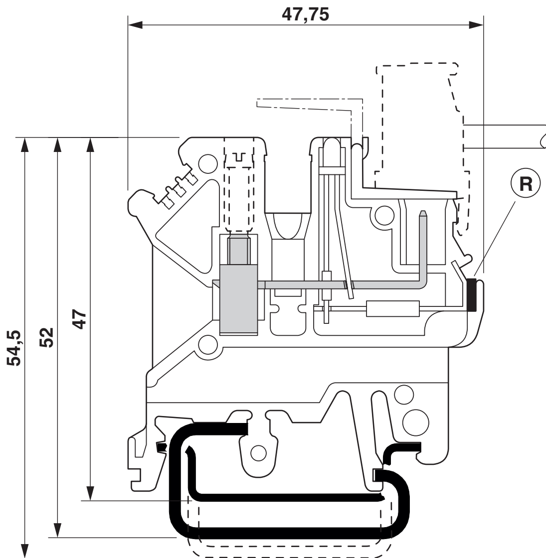
Rysunek wymiarowy
