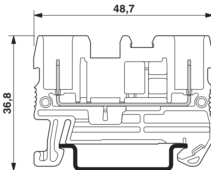
Rysunek wymiarowy
