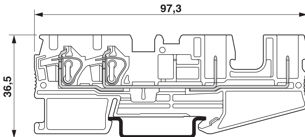
Rysunek wymiarowy
