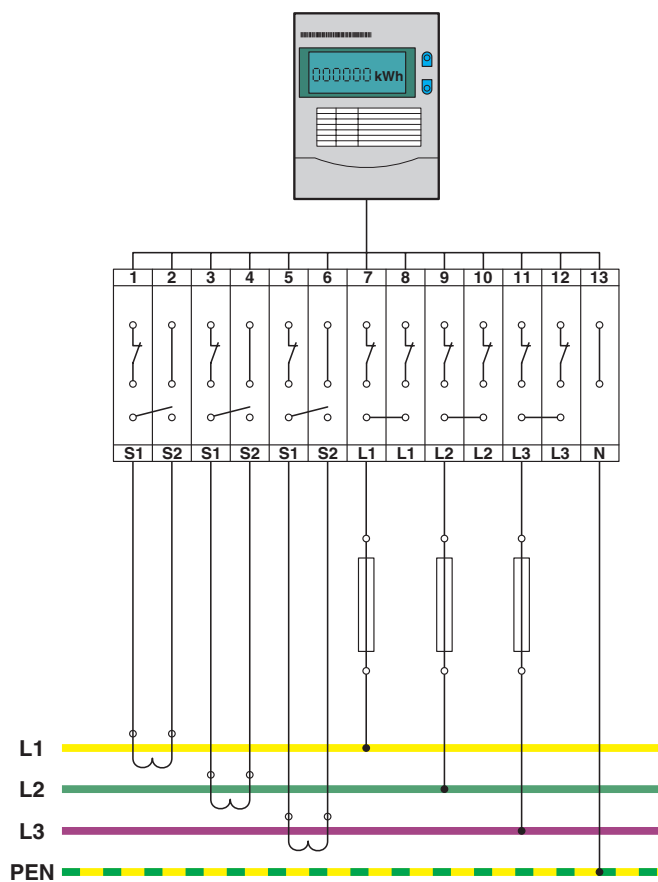
Schemat
