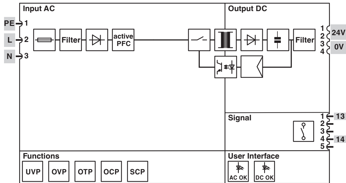
Schemat blokowy
