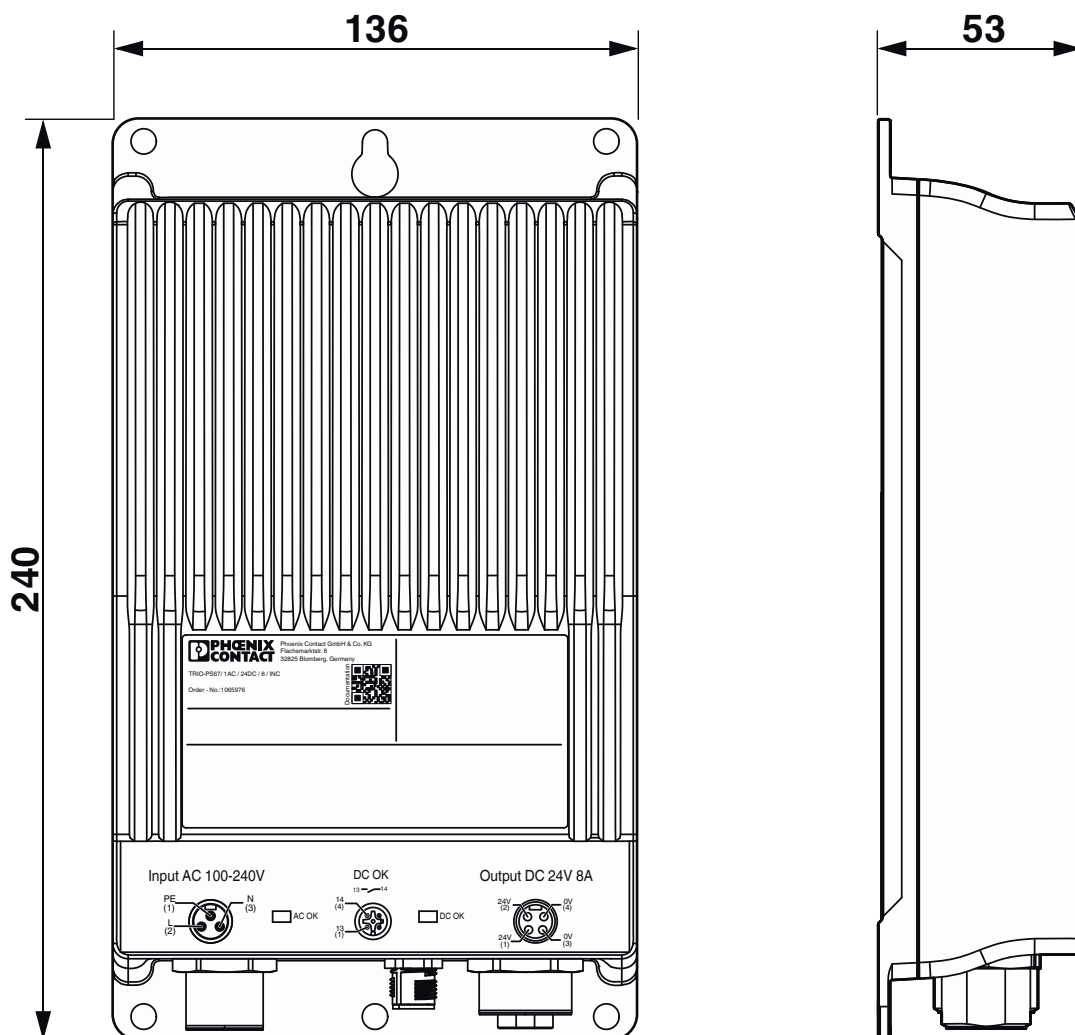
Rysunek wymiarowy
