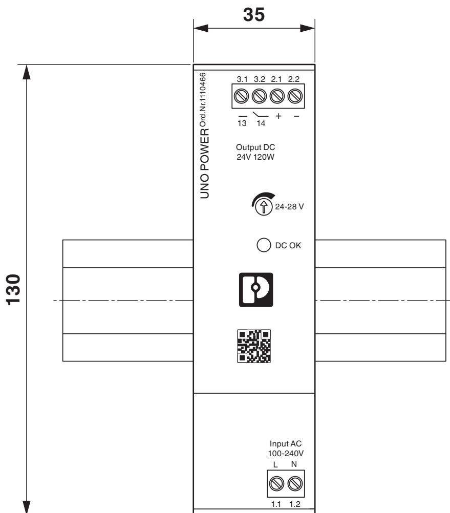
Rysunek wymiarowy
