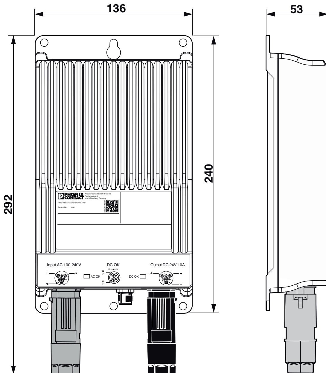
Rysunek wymiarowy
