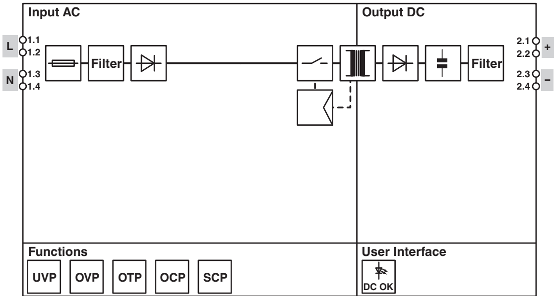
Schemat blokowy
