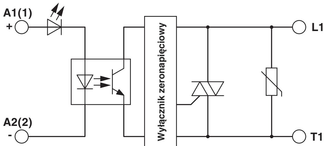
Schemat blokowy
