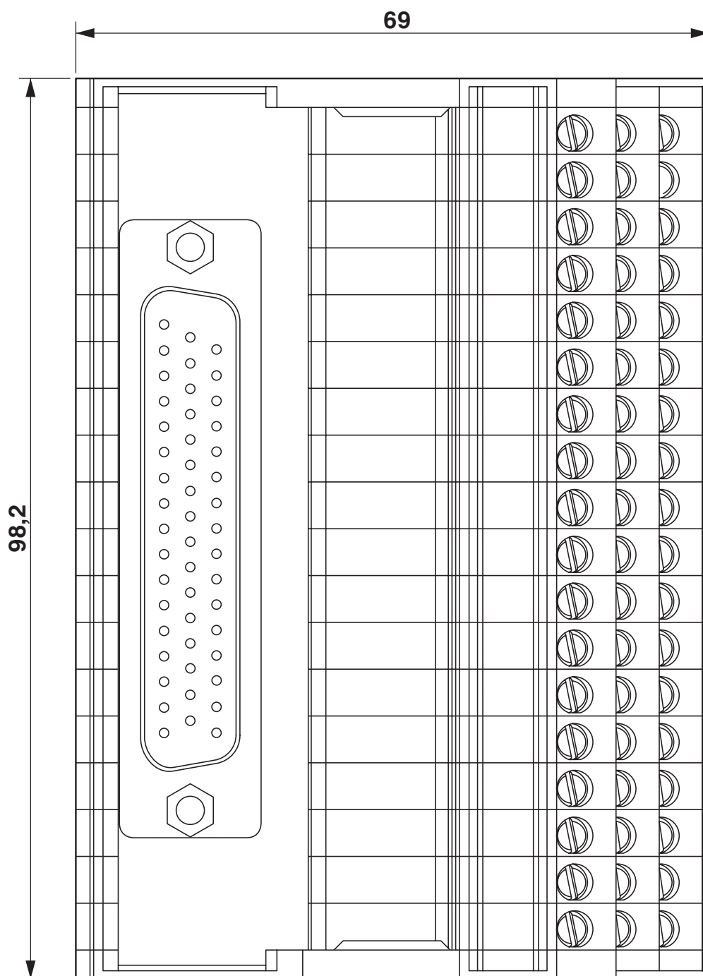
Rysunek wymiarowy
