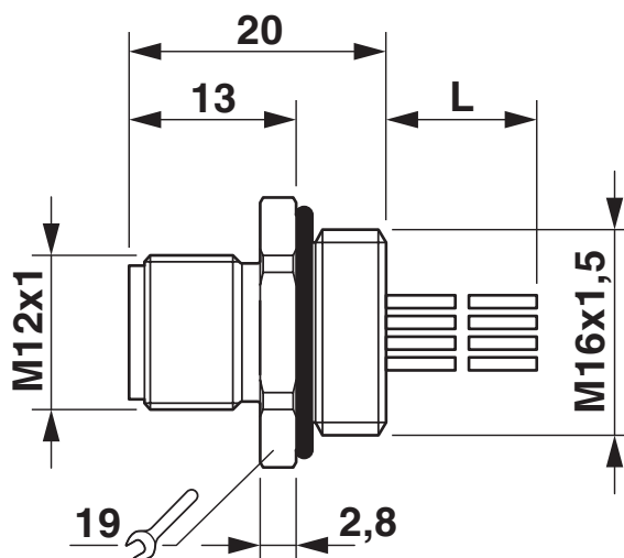
Rysunek wymiarowy
