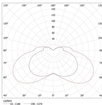
KANLUX S.A. (kat 23104) TERRA LED / Krzywa rozsyłu światła (biegunowo)
