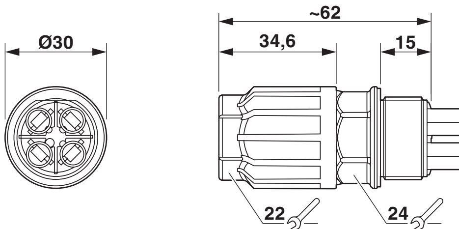
Rysunek wymiarowy
