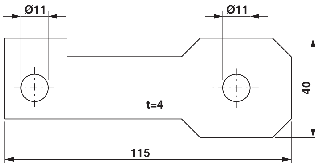
Rysunek wymiarowy
