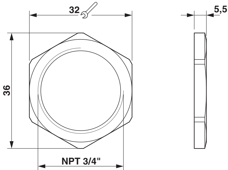
Rysunek wymiarowy
