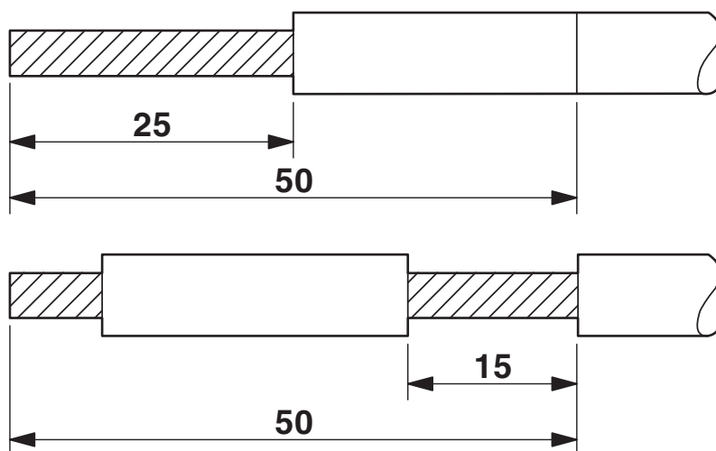
rysunek funkcyjny
