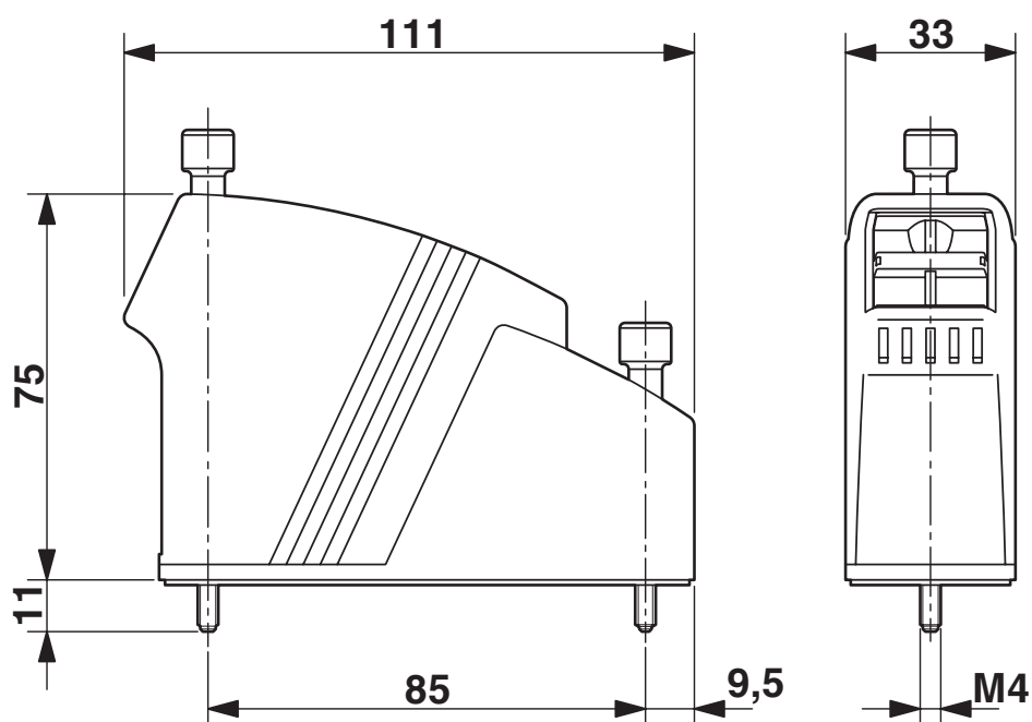
Rysunek wymiarowy
