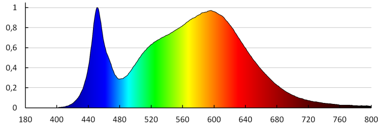
KANLUX S.A. (kat 33751) DULI LED 4W-NW-O-GR / LDC (Polar)
