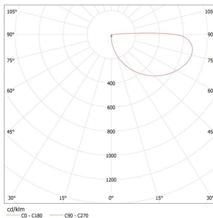
KANLUX S.A. (kat 33751) DULI LED 4W-NW-O-GR / LDC (Polar)
