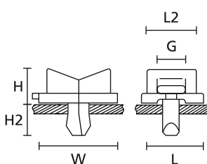
Cokół klinowy TY5K3/5
