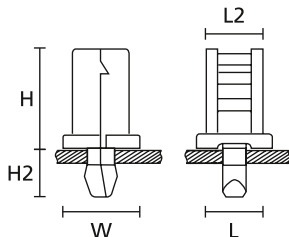
Cokół klinowy TY5K1
