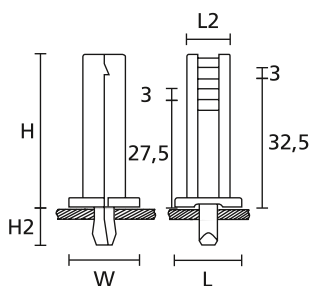
Cokół klinowy TY5K5
