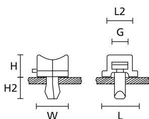
Cokół klinowy TY5K2
