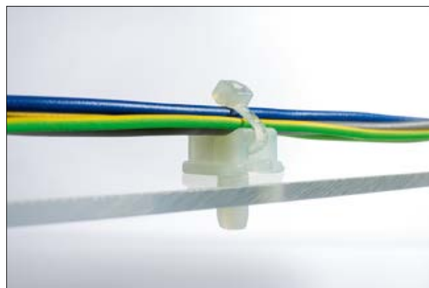
Cokół klinowy TY5, zamontowany.
