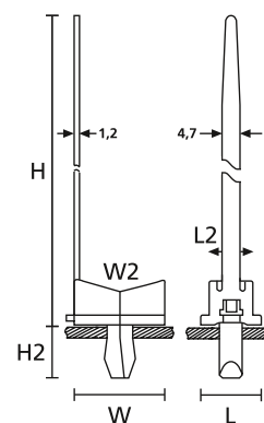
Cokół klinowy TY5K4
