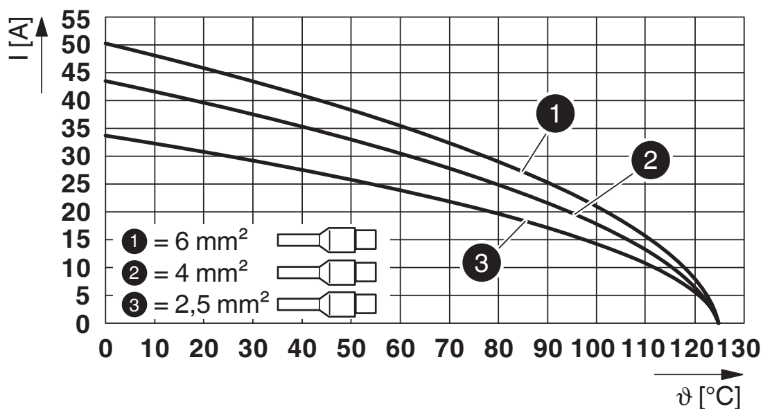
Wykres obniżenia parametrów znamionowych dla linii z tulejką
