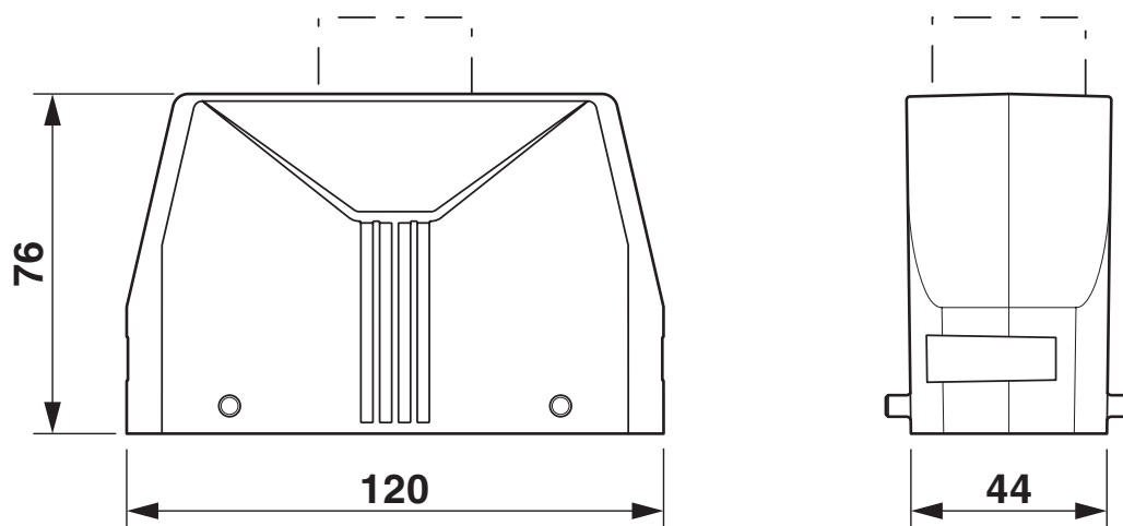
Rysunek wymiarowy
