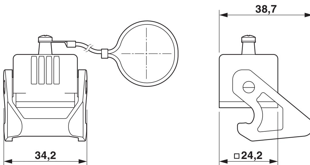
Rysunek wymiarowy
