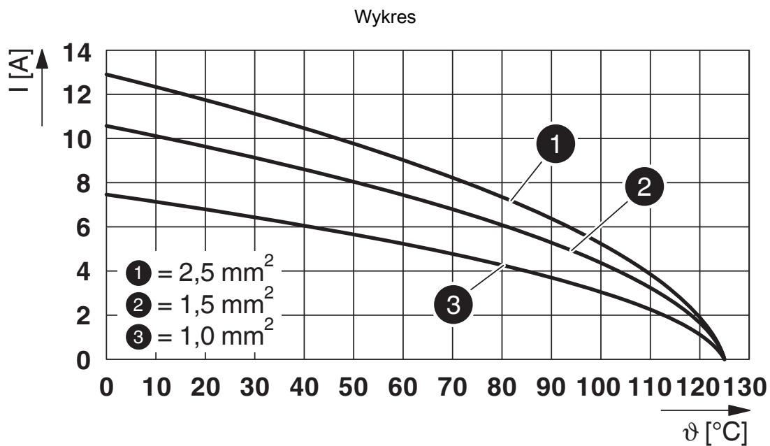
Wykres obniżenia parametrów znamionowych styków toczonego
