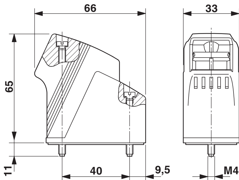
Rysunek wymiarowy
