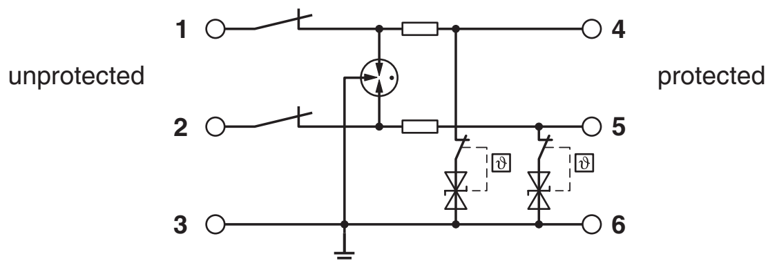
Schemat
