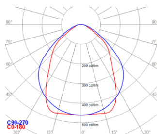
I-LINE 2.0 490_mP_25W
