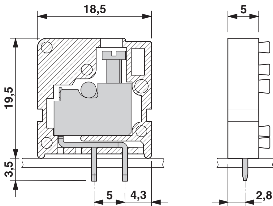
Rysunek wymiarowy
