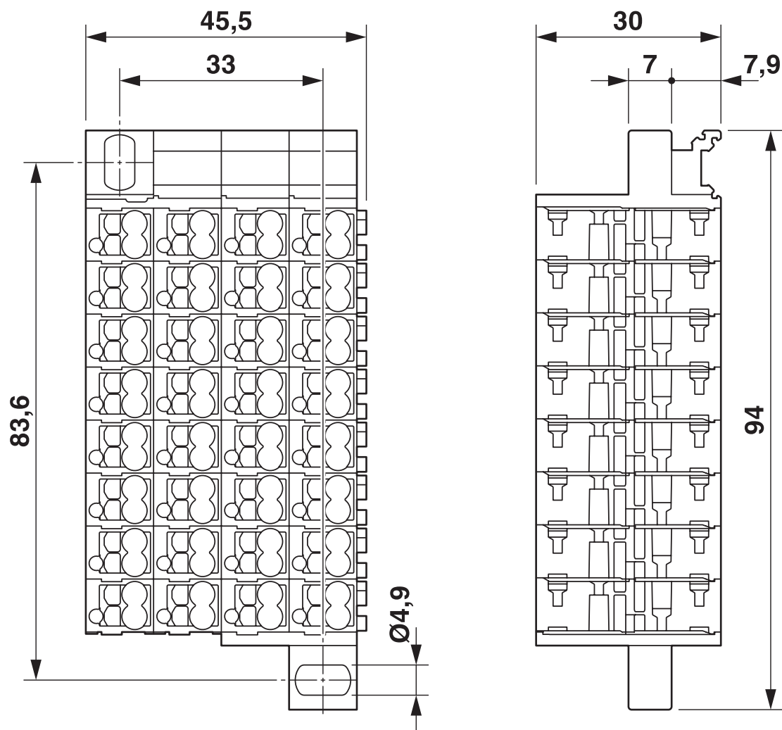
Rysunek wymiarowy
