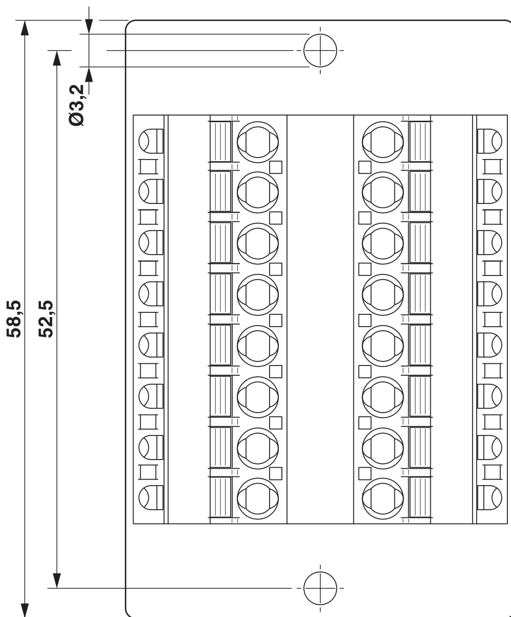
Rysunek wymiarowy
