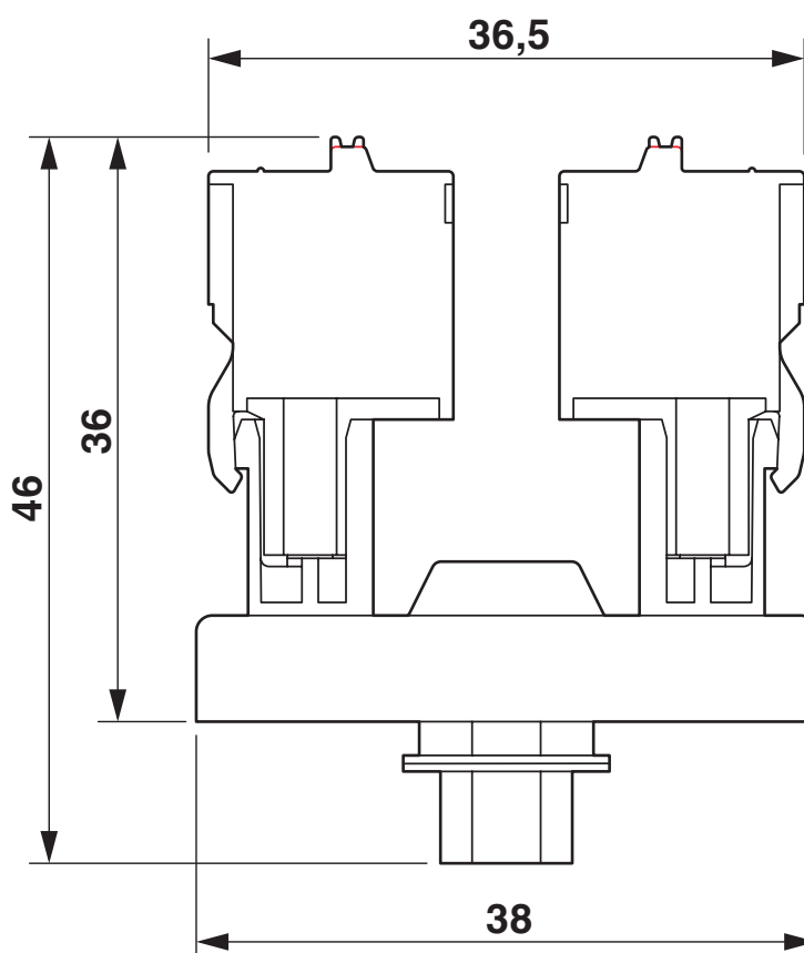
Rysunek wymiarowy
