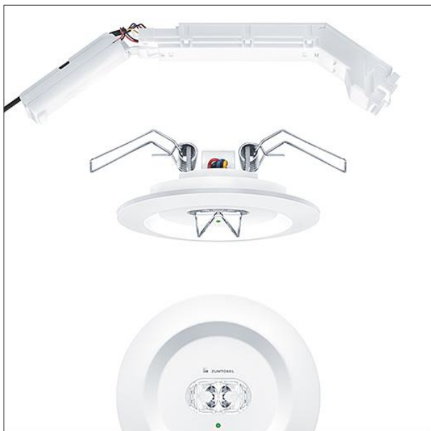
ZS_RES_F_PRO_MRCR_E3D_ESC_WH.jpg
